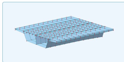
精细化板壳模型
