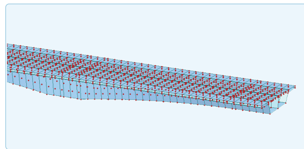
○ 有限元分析模型
