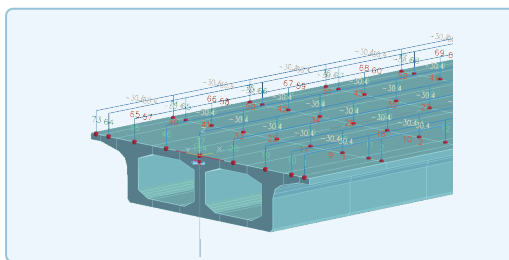
梁格模型
