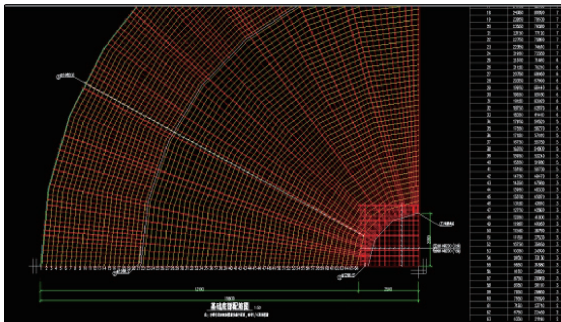
基础底部配筋图
