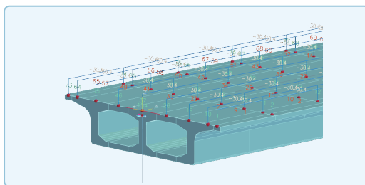
梁格模型
