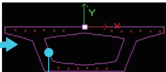
横断面钢筋图
